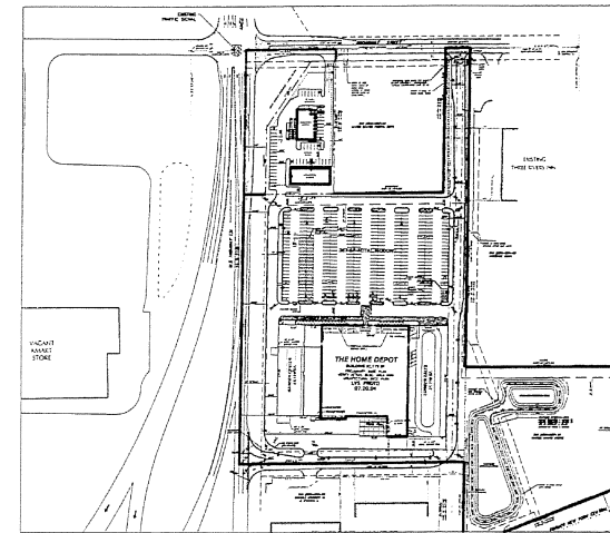
OVERALL SITE (N.T.S.)
